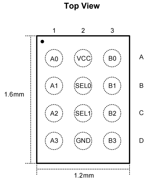
Fig.5-1.GSW550: WLG (WLCSP-12L) Package
