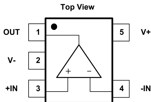
Fig.5-1. GT8551: S5(SOT23-5) Package
