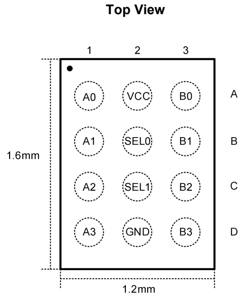
Fig.5-1.GT550: WLG (WLCSP-12L) Package
