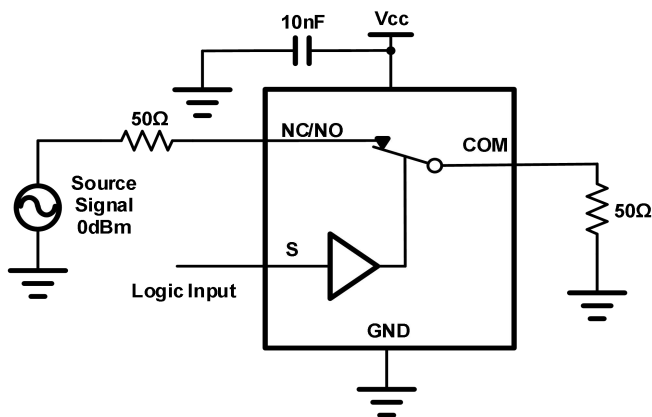
Fig.8-9. Bandwidth
